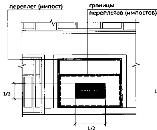
1/2 высоты и ширины расстояния между импостами
